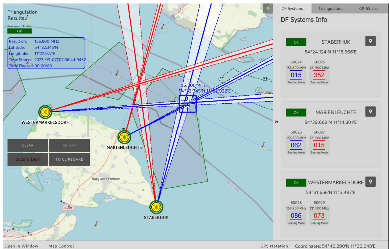
Abbildung 72: Nur Triangulationsergebnisse innerhalb der Polygone sind gültig
