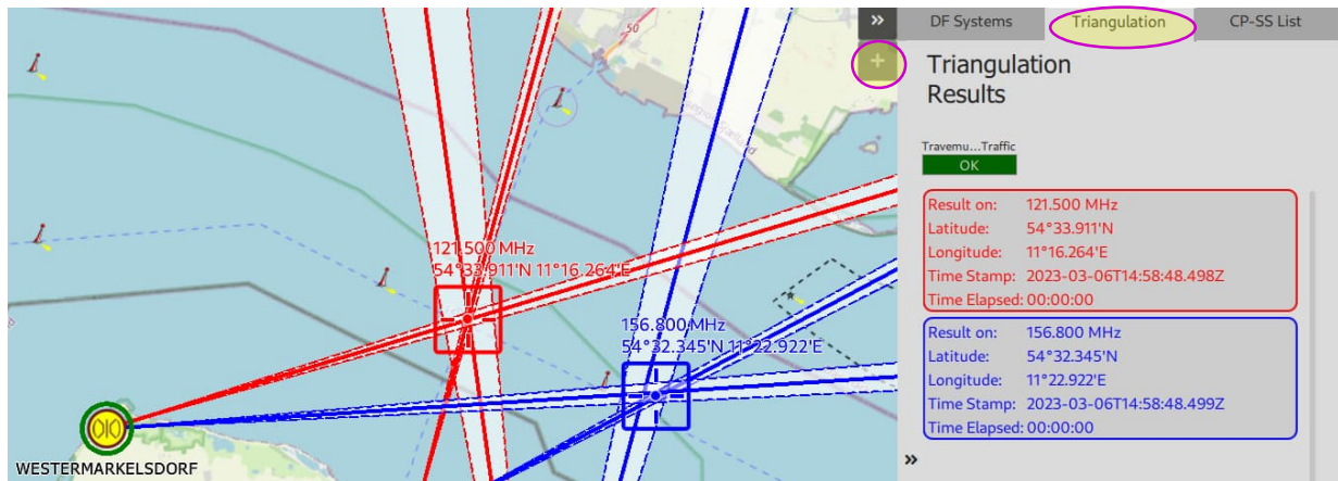
Abbildung 66: Numerische Triangulationsergebnisse in der Seitenleiste
