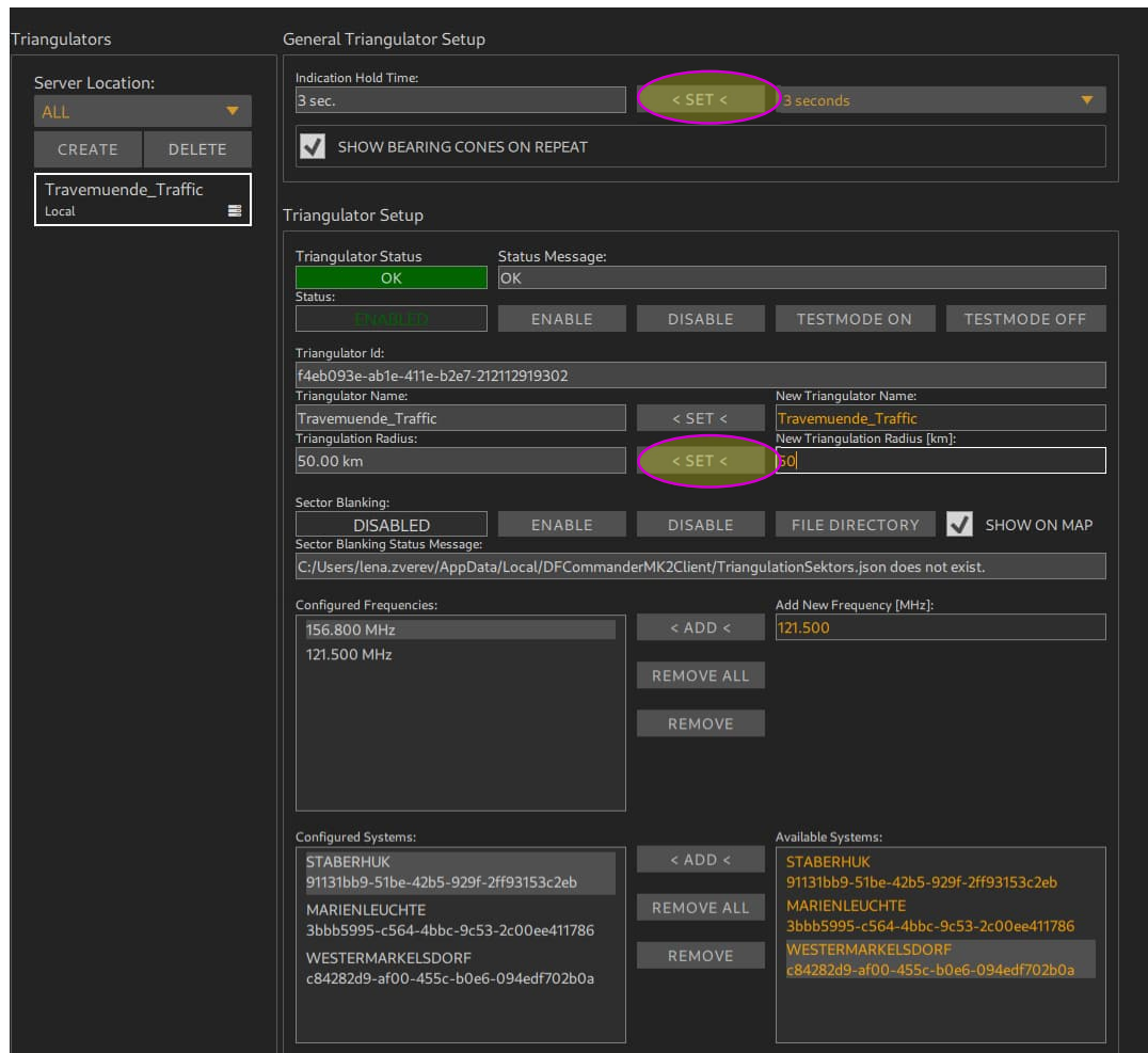
Abbildung 63: Triangulator erfolgreich eingestellt
