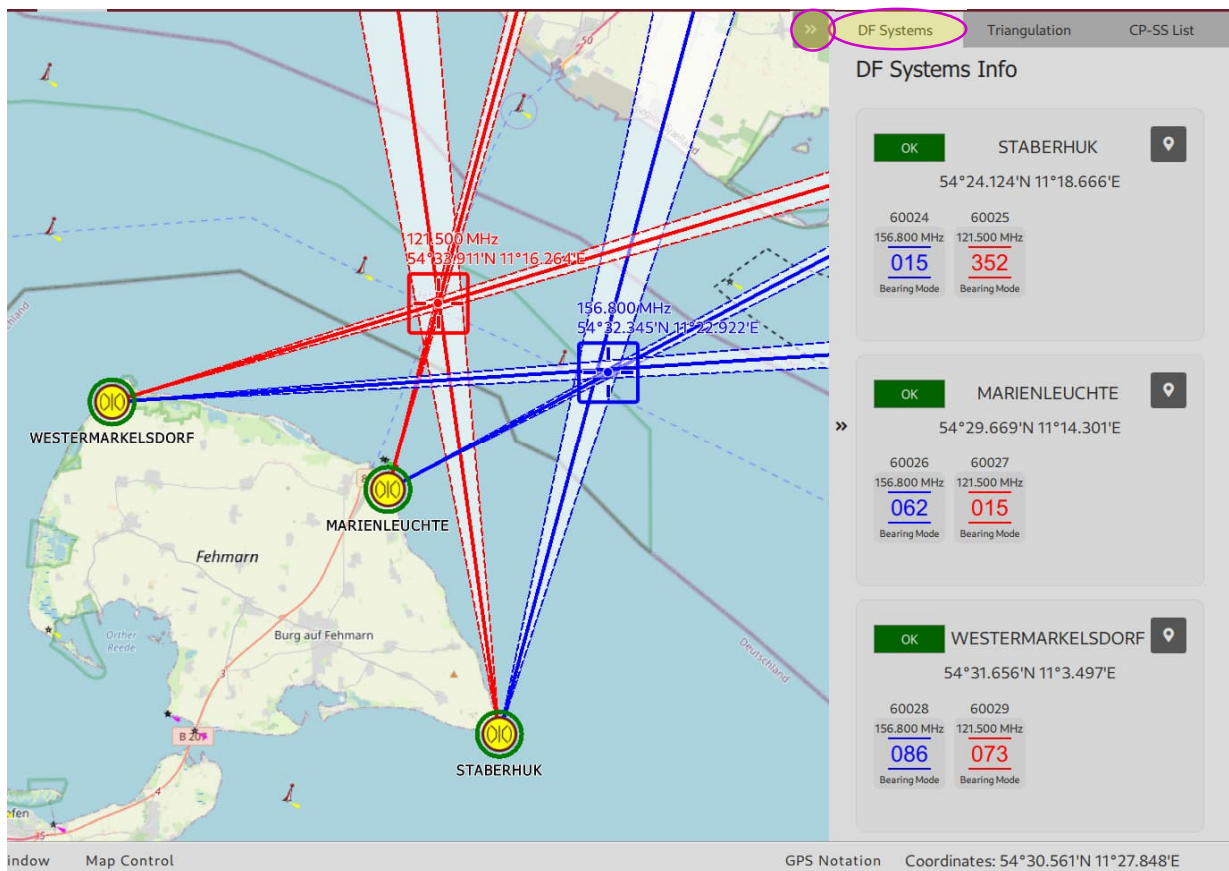
Abbildung 65: Triangulationsergebnisse auf der Karte
