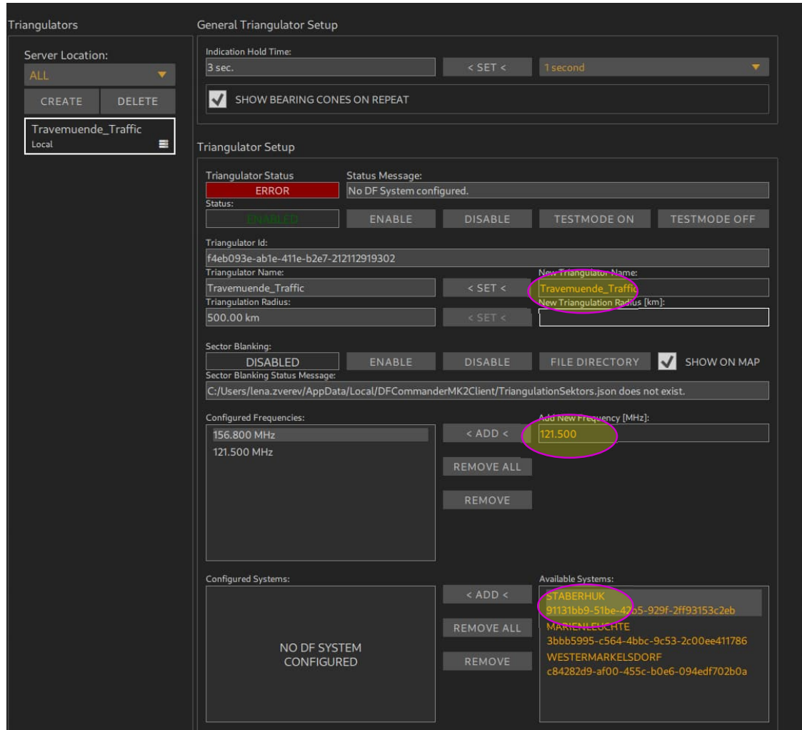
Abbildung 62: Triangulator Frequenzeinstellung
