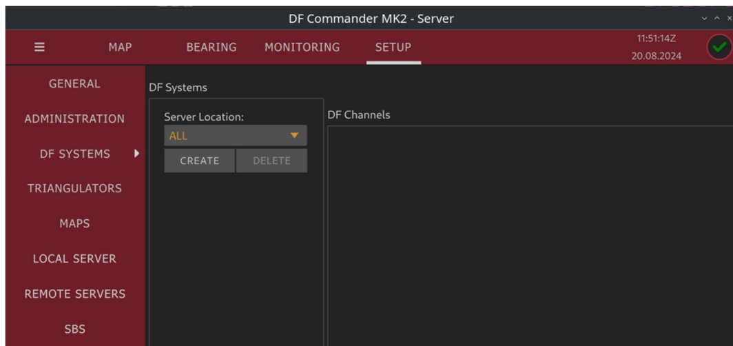
Abbildung 22: Leere Systemliste
