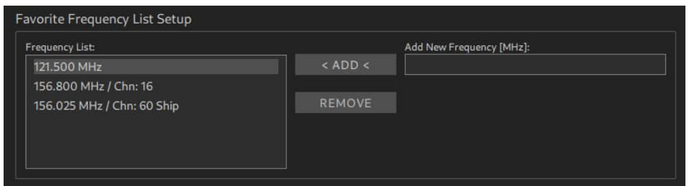
Abbildung 12: Frequenzfavoritenliste
