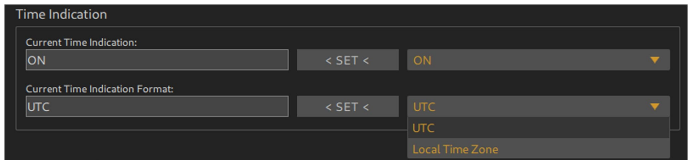
Abbildung 10 Zeitanzeige-Formatoptionen
