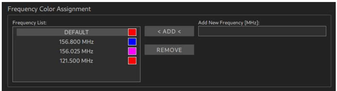
Abbildung 11: Frequenz-Farbzuzuweisung
