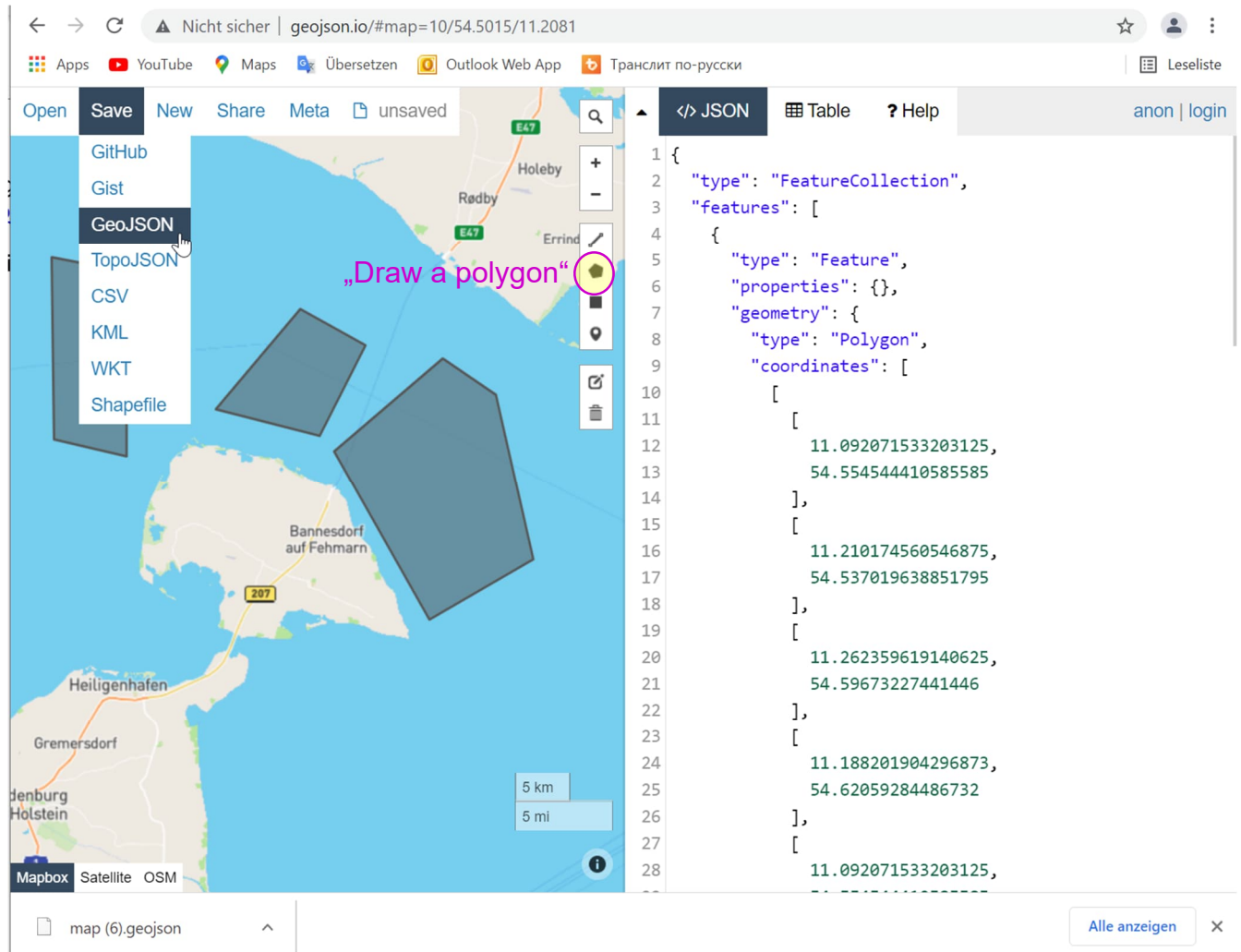
Abbildung 70: www.geojson.io
