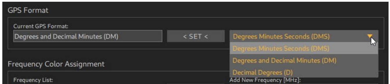
Abbildung 9: GPS-Format
