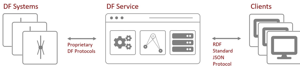
Abbildung 3: DF-Service
