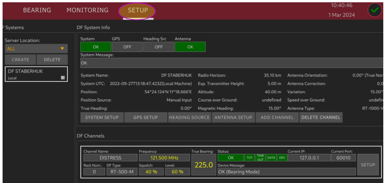
Abbildung 56: Überprüfung im SETUP Menu
