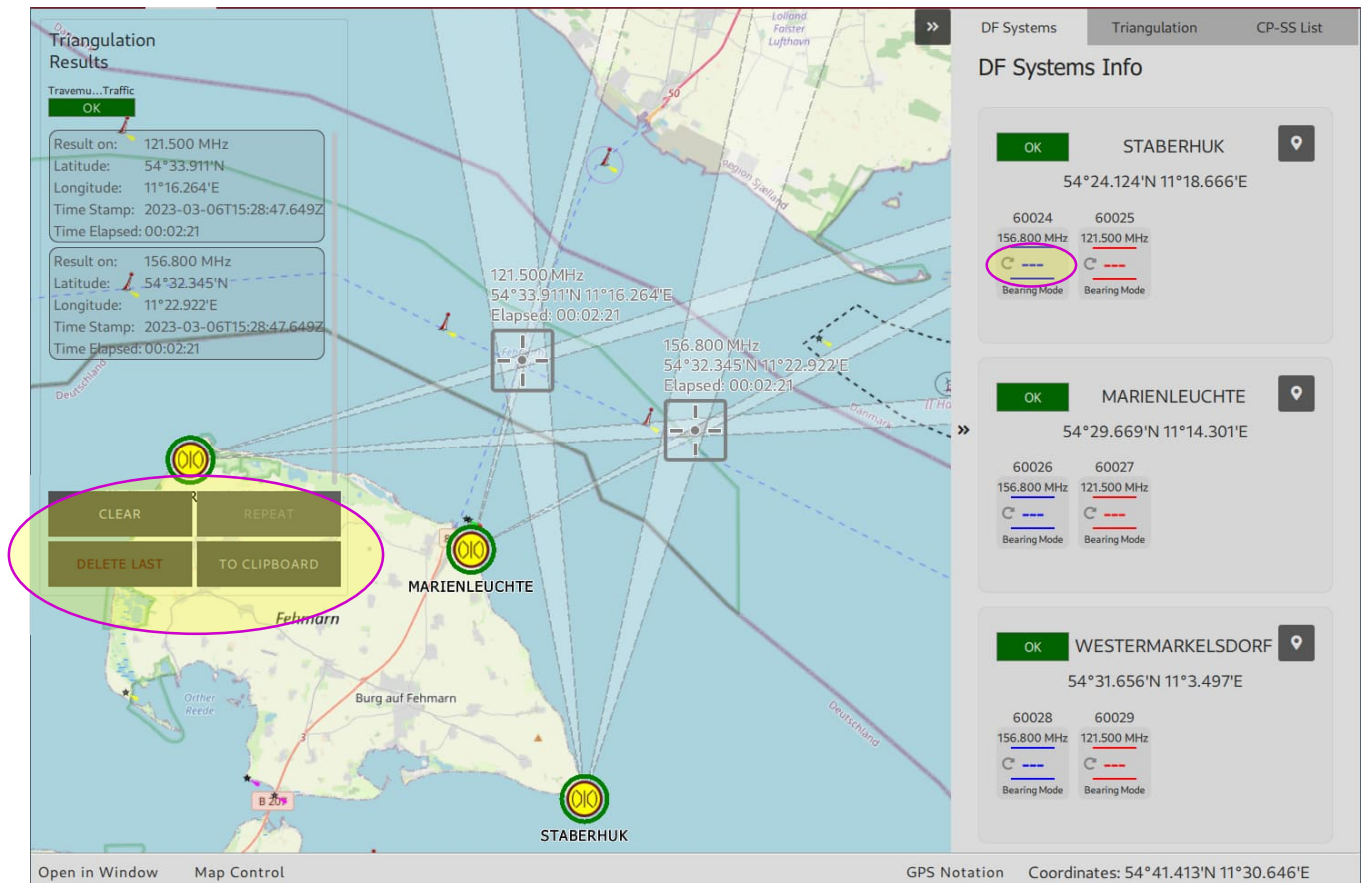
Abbildung 68: REPEAT und CLEAR
