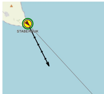
Abbildung 25: Das mobile DF-System verwendet den COG-Wert des GPS-Geräts und den Kurswert des Kursquellgeräts
