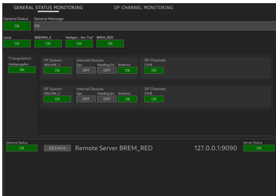
Abbildung 85: Anzeige des redundanten Servers auf der Monitoring Page
