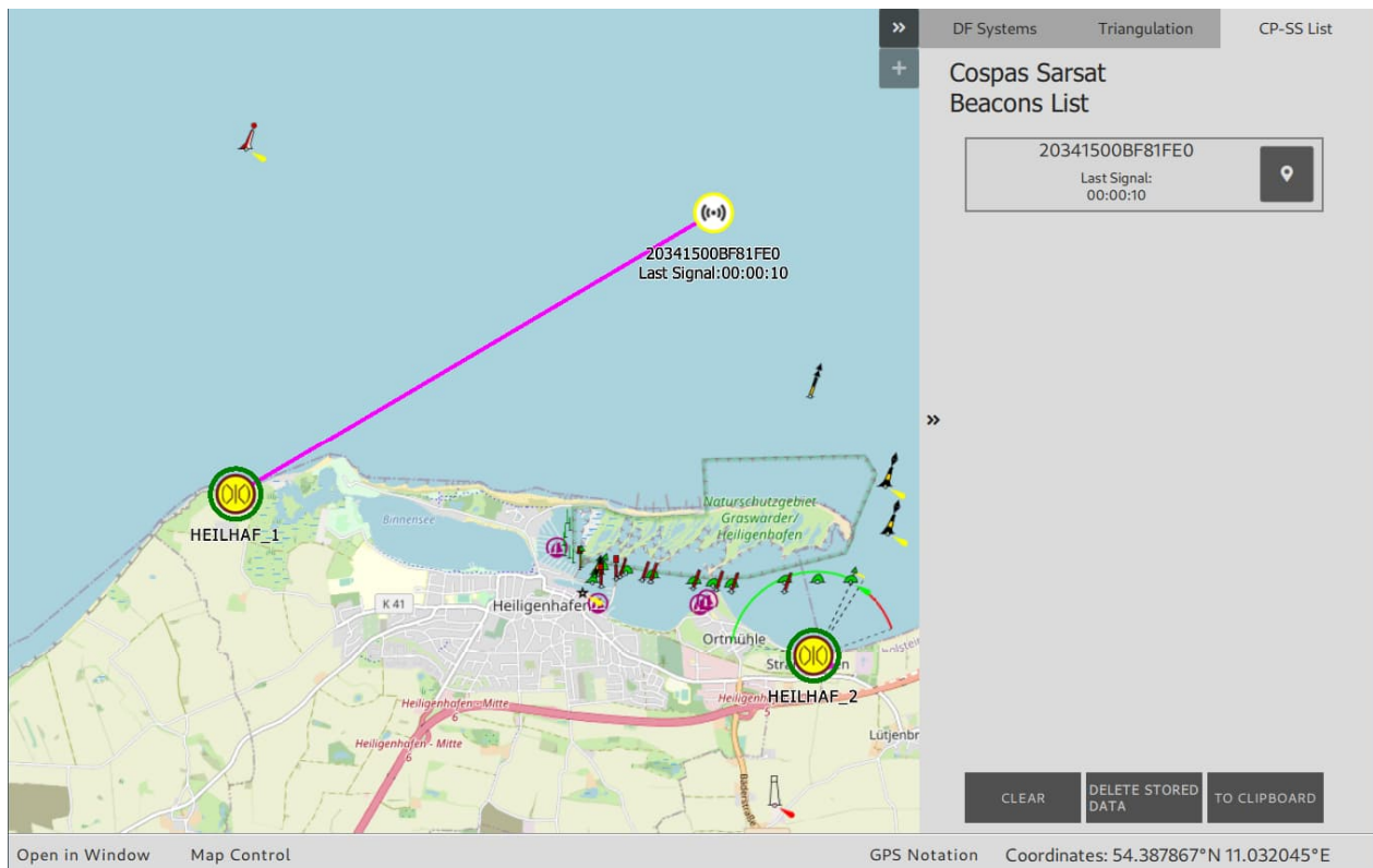
Abbildung 102: Dekodierendes Peilsystems mit der Peillinie zum CP-SS-Beacon
