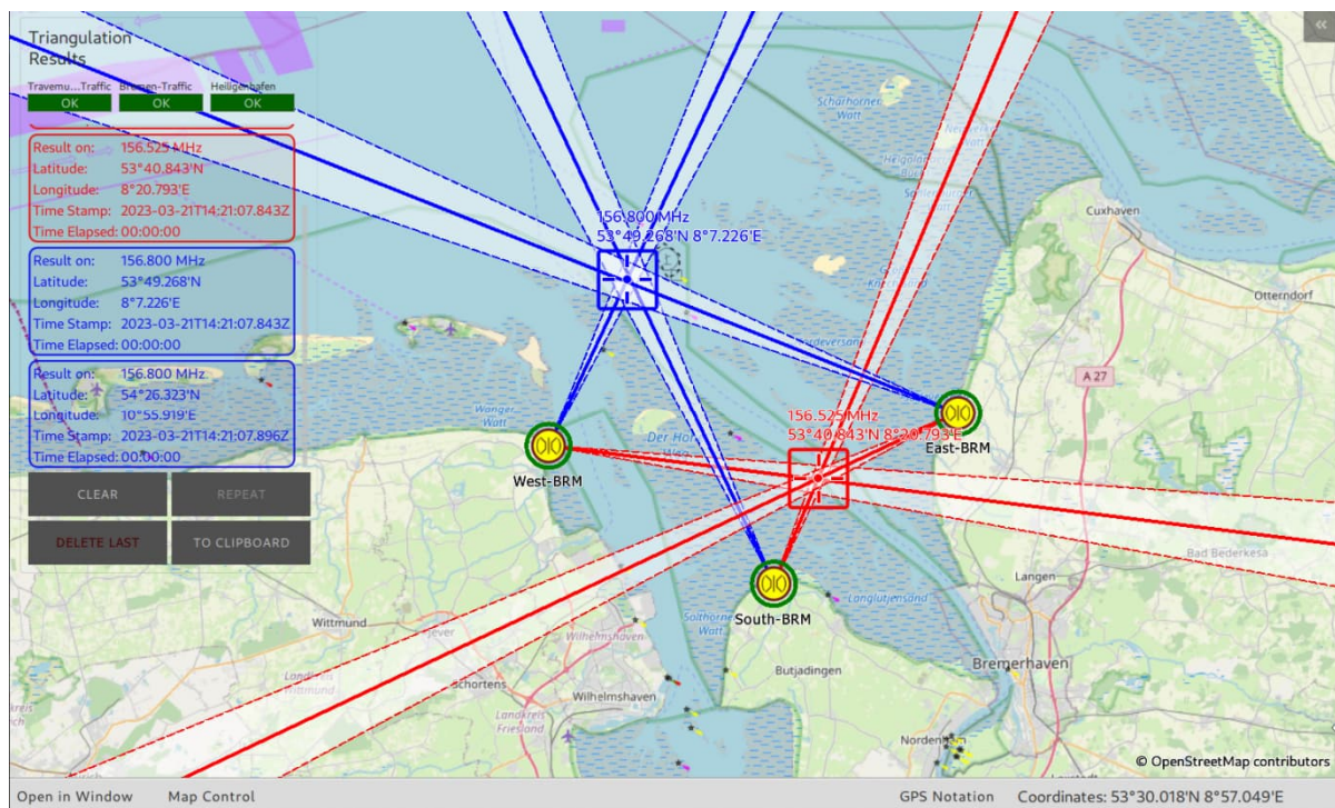
Abbildung 81: Remote Server auf der MAP Page
