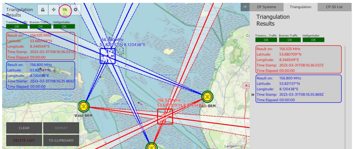
Abbildung 67: Numerische Triangulationsergebnisse in dem separaten Fenster
