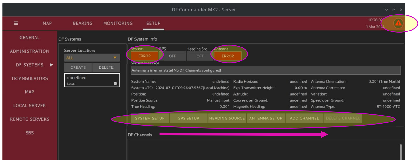
Abbildung 23: Neues DF-System
