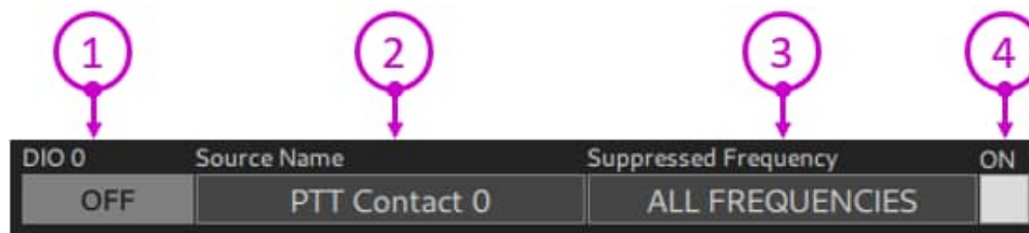
Abbildung 91: DIO Setup
