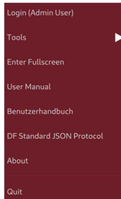
Abbildung 5 Drop-down Menu
