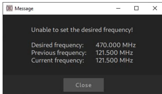
Abbildung 55: Fehlermeldung Frequenz
