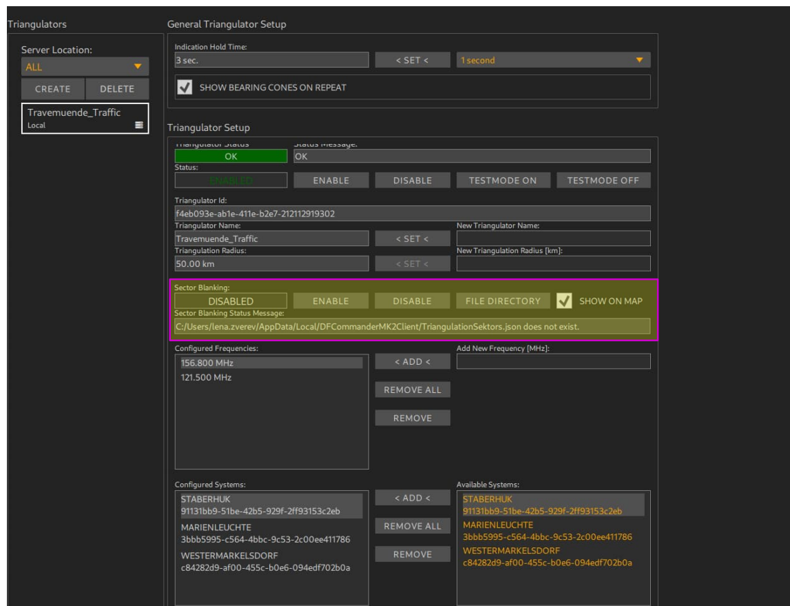
Abbildung 69: Sector Blanking
