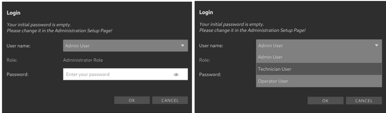
Abbildung 18 Anmeldedialog
