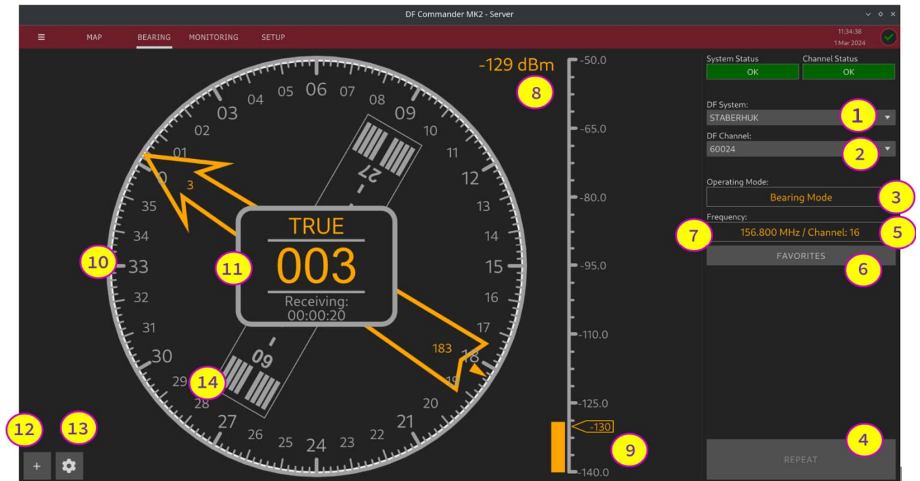
Abbildung 98: Bearing Page
