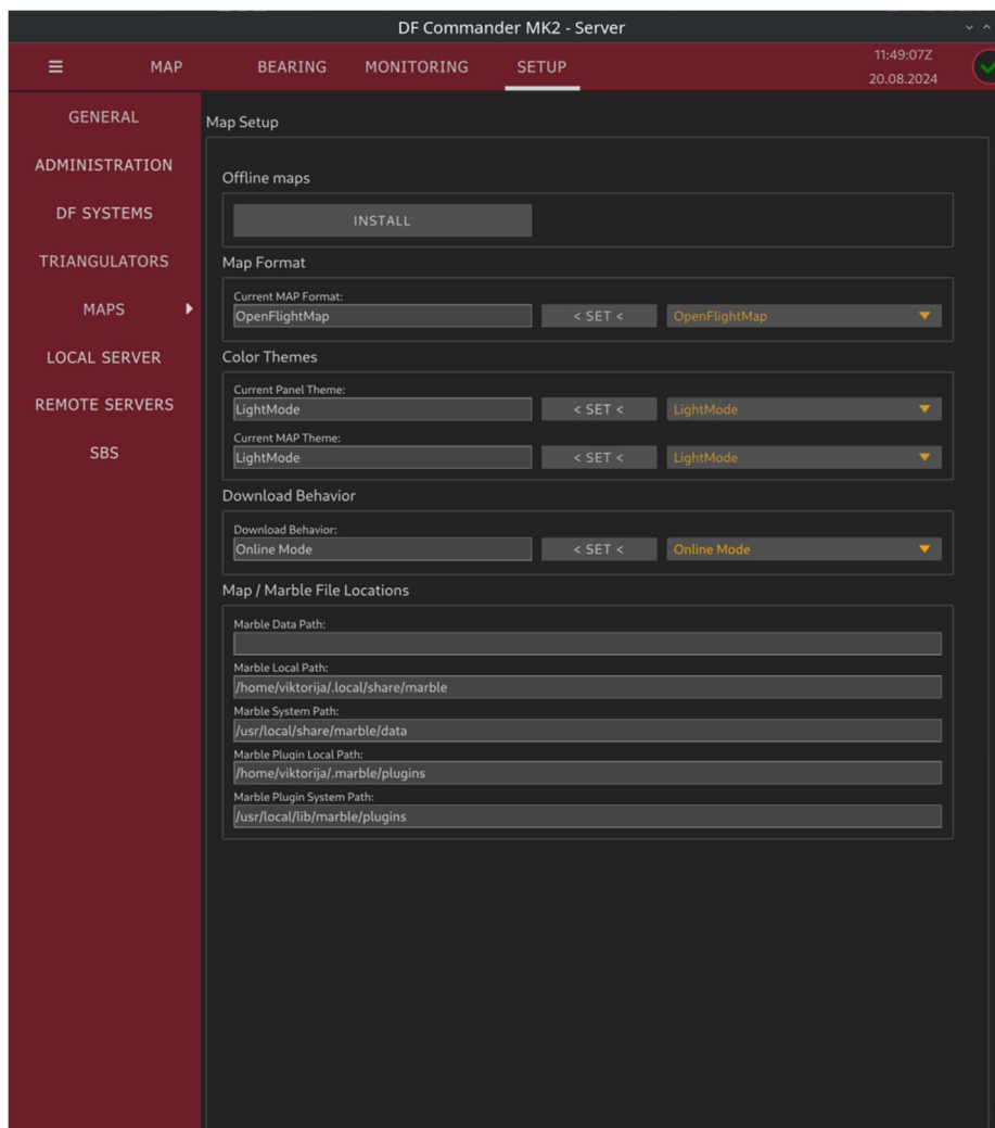
Abbildung 21: MAP SETUP
