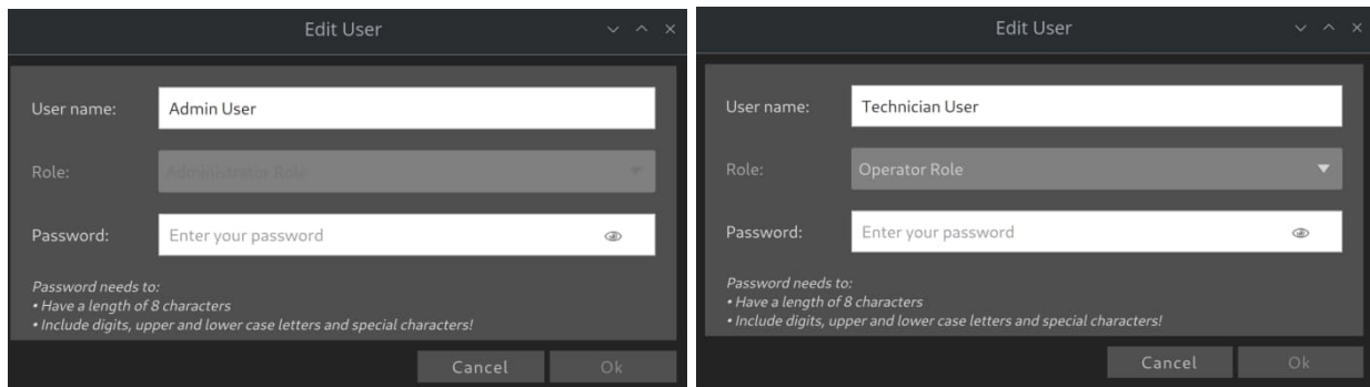
Abbildung 16 User Dialog
