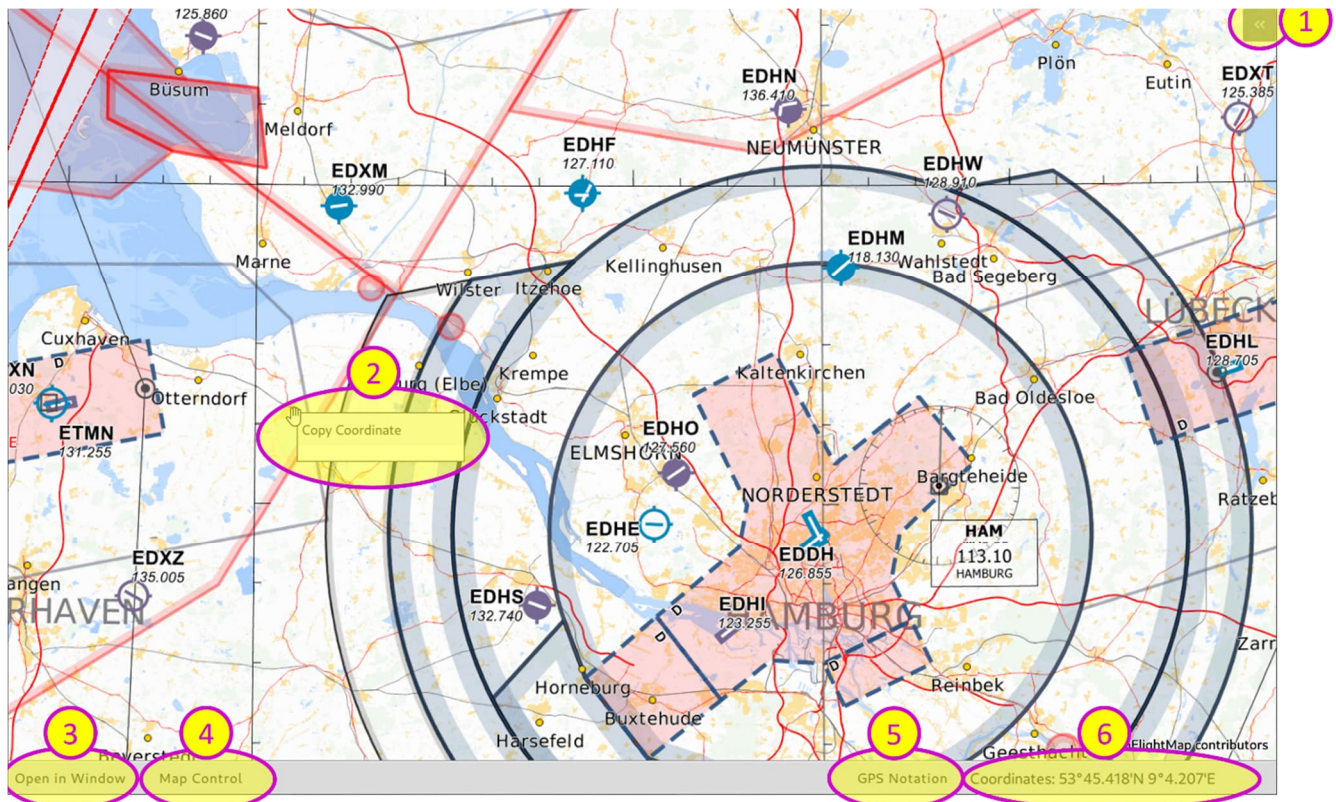
Abbildung 100: Kartenanzeige
