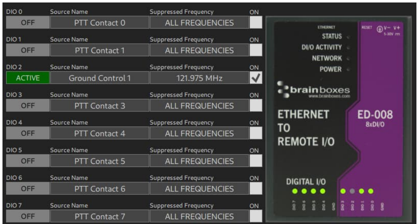
Abbildung 92: SBS-Beispiel
