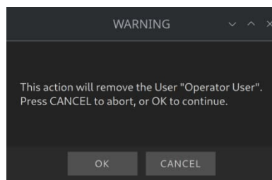
Abbildung 17 Löschbestätigung
