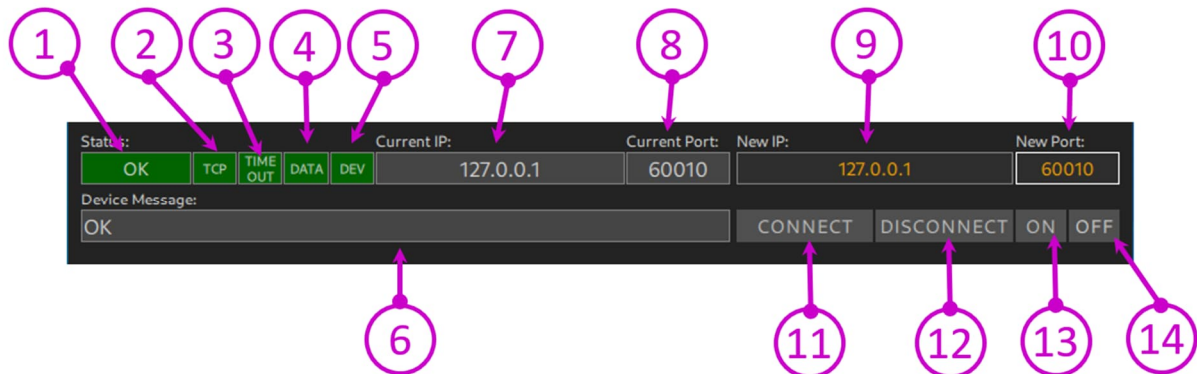
Abbildung 93: Status Anzeigen
